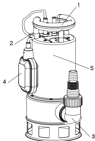
Рис. 1. Внешний вид.
