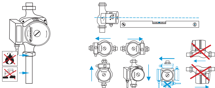
Рисунок 3. Правила установки насоса
