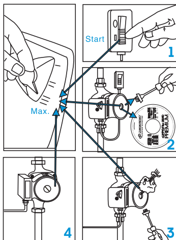
Рисунок 5. Схема выпуска воздуха
