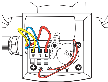
Рисунок 4. Схема электрического подключения
