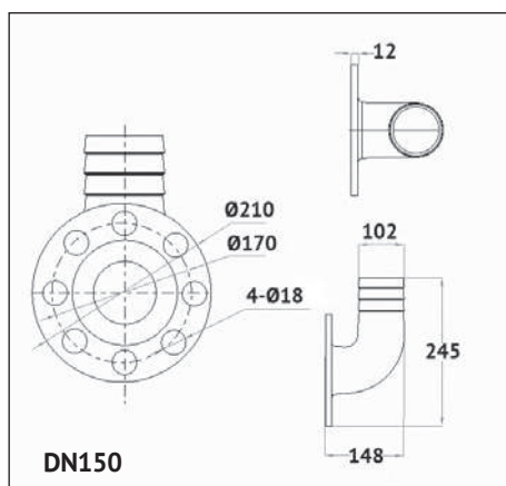
Рисунок 2 – Габаритные и присоединительные размеры углового переходника-адаптера
